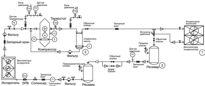
Рисунок 2 – Схема фреонового промышленного кондиционера
